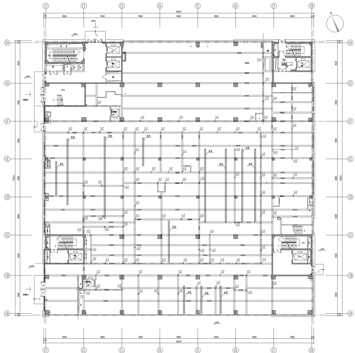
后勤综合楼一层架空层地垄墙、构造柱、水沟示意图
